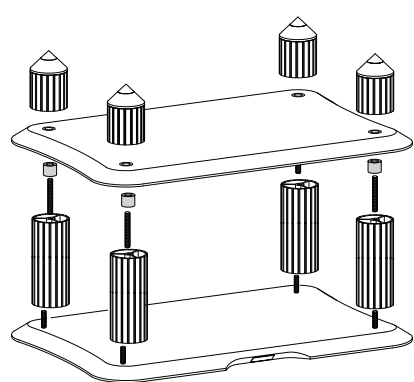
БАЗОВАЯ СТОЙКА (С ДВУМЯ ПОЛКАМИ)
