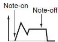
Ноты берутся с большой velocity; "At", "Dc", "St" и "RI" установлены в "-"
