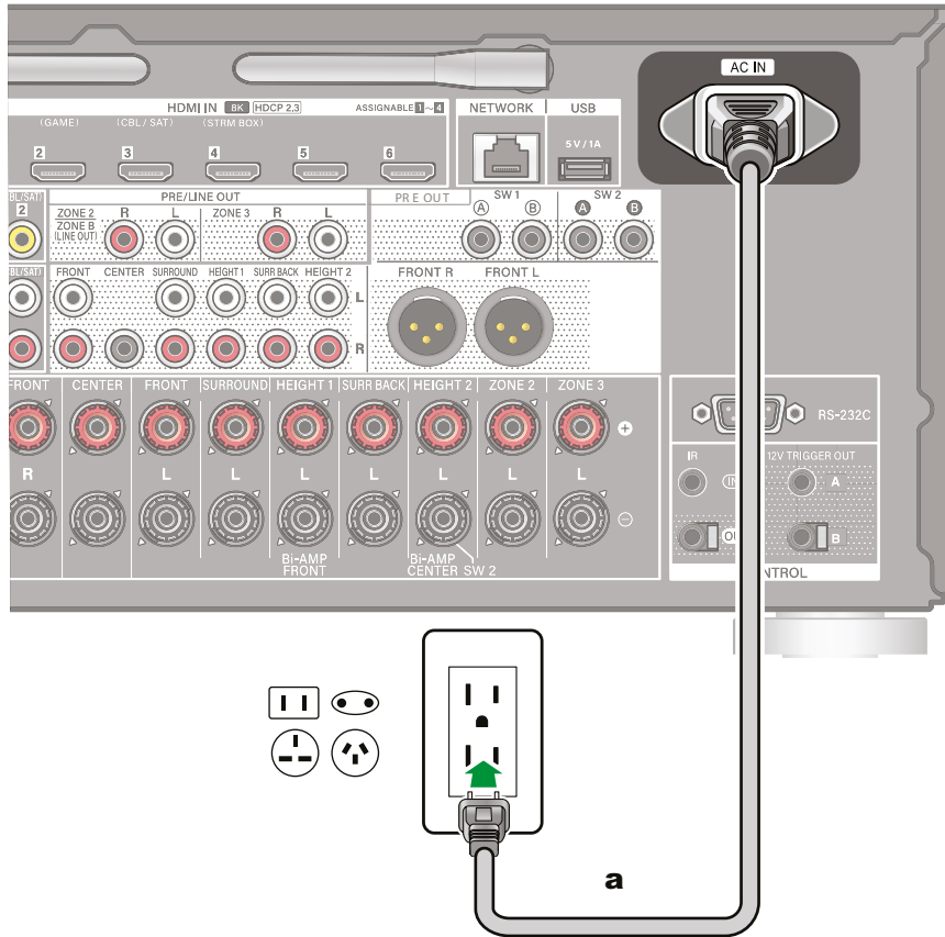
a Шнур питания
