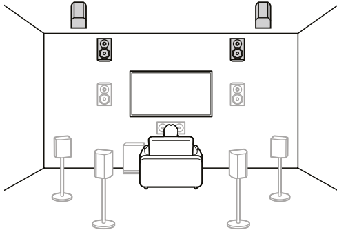
7.1.4-канальная конфигурация (фронтальные верхние и тыловые верхние) ( → стр. 38 )
