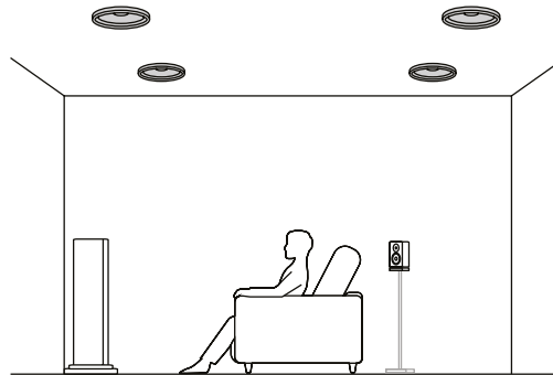
5.1.4-канальная конфигурация (потолочные фронтальные и потолочные тыловые) ( → стр. 37 )
