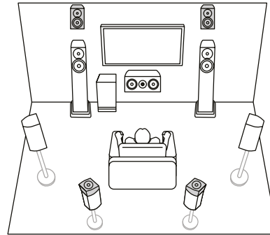
7.1.4-канальная конфигурация (фронтальные верхние и АС с поддержкой Dolby (тыловые окружающие)) ( → стр. 38 )
