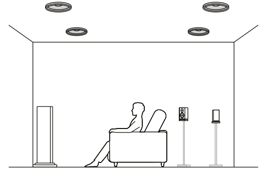
7.1.4-канальная конфигурация (фронтальные и тыловые потолочные) ( → стр. 38 )
