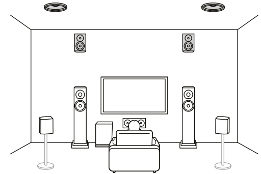
5.1.4-канальная конфигурация (фронтальные верхние и тыловые потолочные) ( → стр. 37 )
